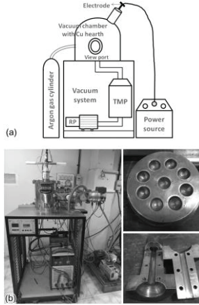
Şekil 3.4 (a) Vakum arklı eritme ünitesinin şeması ve (b) bakır pota ve iki tip bakır kalıp içeren ark eritme ve emme döküm ekipmanının fotoğrafı
