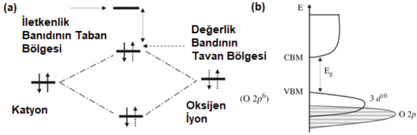
Şekil 2.2: Bakır tabanlı oksitlerin band diyagramı. a) Oksijen iyonları ve katyonlar arası kimyasal bağlar. b) Metal ve oksijen enerji seviyeleri [Crepelliere et al, 2016].
