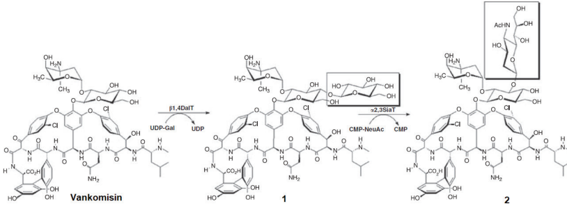
Şekil 12. Vankomisin \beta 1,4GalT enzimiyle elde edilen türevi (1) ve \alpha 2,3-SiaT enzimiyle elde edilen türevi (2)
