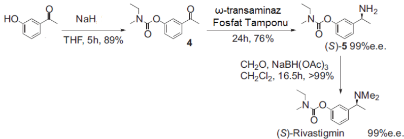
Şekil 14. Paracoccus denitrificans kaynaklı transaminaz enzimi ile (S)-rivastigmin sentezinin basamakları (Fuchs ve diğerleri, 2012: 7692)
