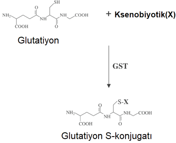
Şekil 5. Ksenobiyotiğin glutatiyon S-konjugatına dönüşümünü katalizleyen Glutatiyon-S-transferazın (EC 2.5.1.18) tepkimesi (Townsend ve Tew, 2003: 7370)
