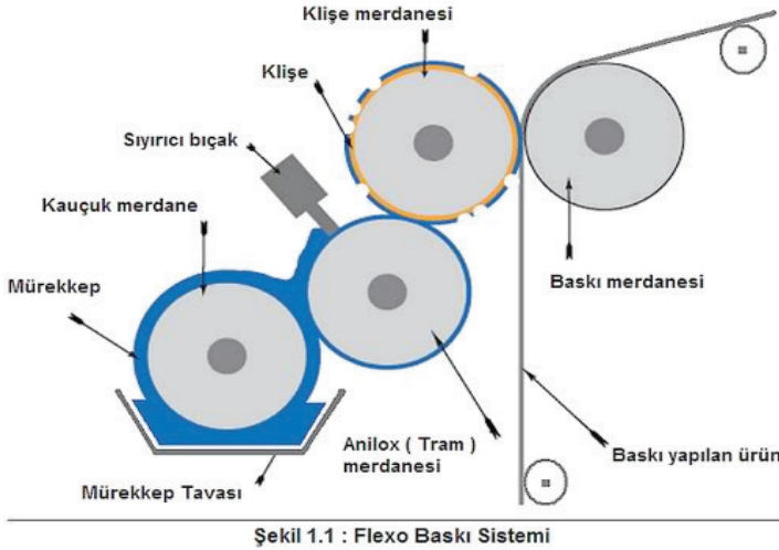
Şekil 1.1 : Flexo Baskı Sistemi
