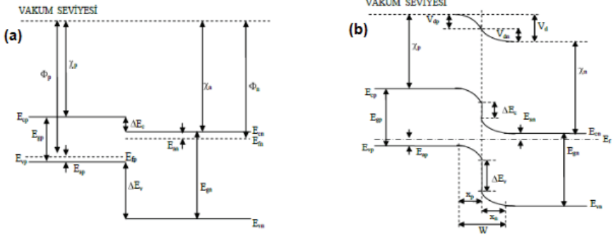
Şekil 2.5: a) Yalıtılmış iki farklı yarıiletkenin eklem oluşturmada önceki bant yapısı, b) Eklem oluştuktan sonraki bant yapısı (Isısal dengede) [Kitai, 2011].
