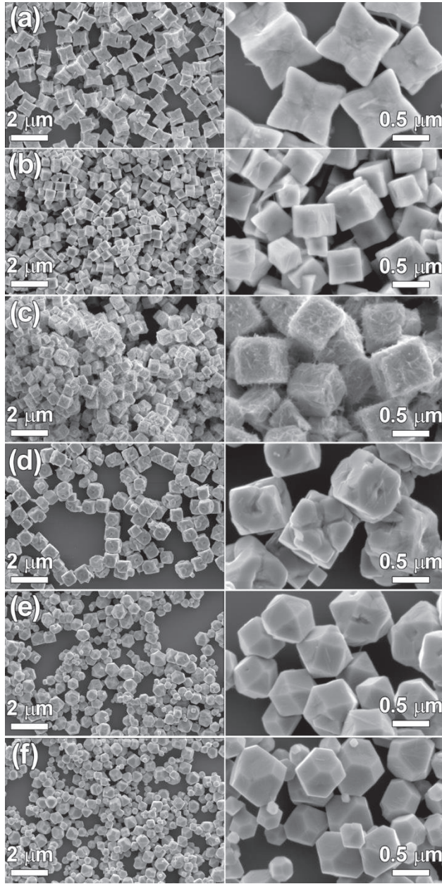
Şekil 2.4: \text{Cu}_2\text{O} ürünlerinin morfolojik özelliklerinin karşılaştırılması. Temsili düşük (sol panel) ve yüksek (sağ panel) büyütme SEM görüntüleri, reaksiyona eklenen farklı miktarlarda \text{NH}_2\text{OH}.\text{HCl} ile hazırlanan \text{Cu}_2\text{O} örneklerini göstermektedir: a) 35, b) 45, c) 55, d) 65, e) 85 ve f) 125 mL. [Argibay et al., 2015].
