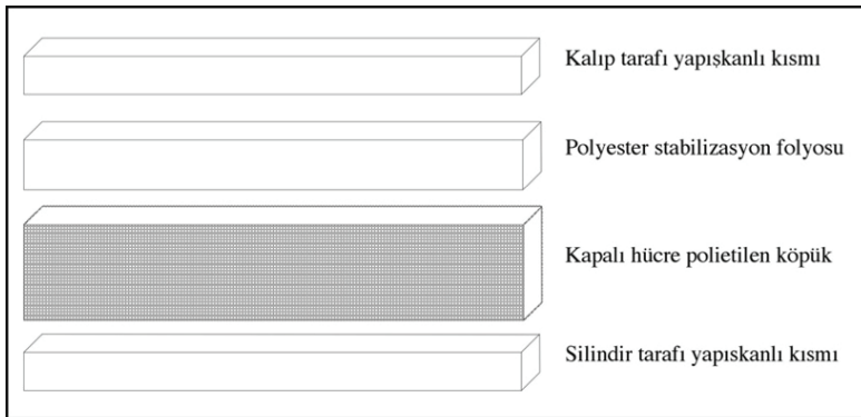
Şekil 7. Yapıştırma bant katmanları
