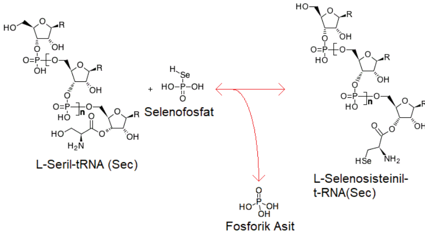
Şekil 9. L-seril-tRNA Sec selenyum transferazın (EC 2.9.1.1) katalizlediği bir tepkime (“Orthology: K01042”, t.y.)
