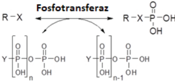
Şekil 7. Fosfotransferazların katalizlediği bir tepkime örneği ("Phosphotransferases", t.y.)
