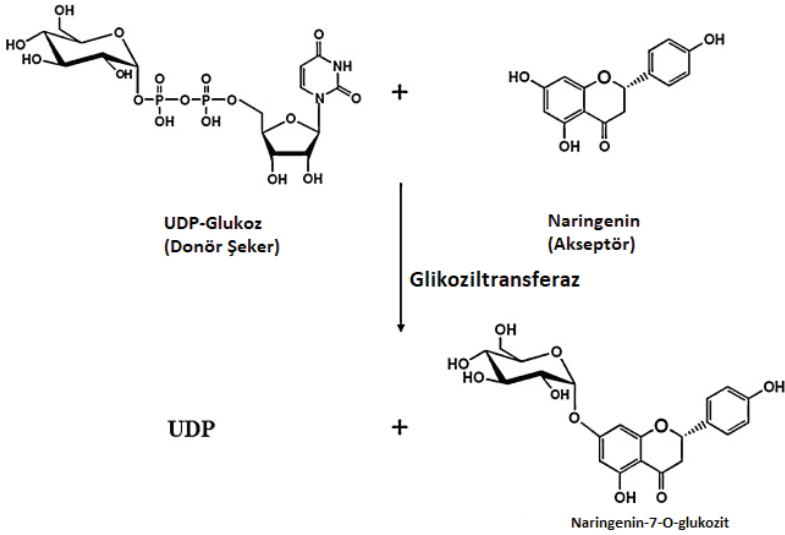
Şekil 4. Glikoziltransferazın katalizlediği bir tepkime örneği (Choi, Kim, Yoon, Kim ve Lee, 2012)
