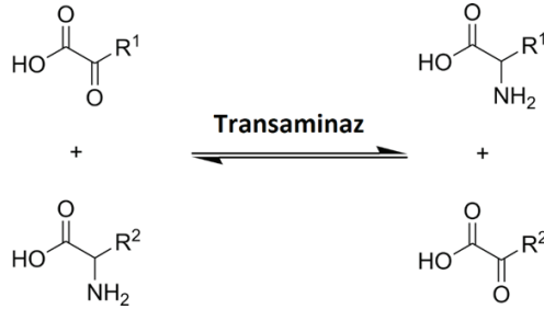
Şekil 6. Transaminazların katalizlediği bir tepkime örneği (Transaminase, t.y.)
