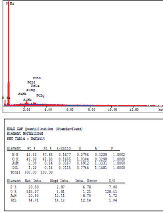
Şekil 7. \text{LiB}_3\text{O}_5 bileşiğinin EDX grafiği
