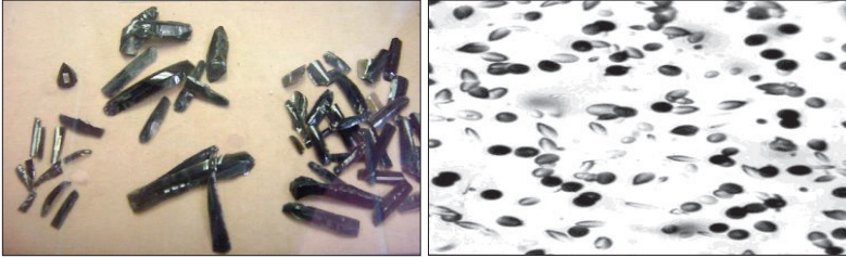
Şekil 7. (a) Kullanım için hazırlanmış obsidiyen malzemeler, (b) fizyon izleri (Göksu ve ark., 1991).
