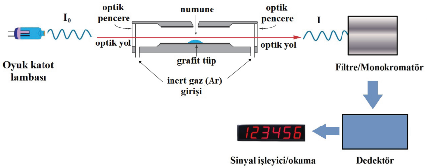
Şekil 8. Elektro Termal/Gratit Fırınılı Atomik Absorpsiyon Spektrometresi
