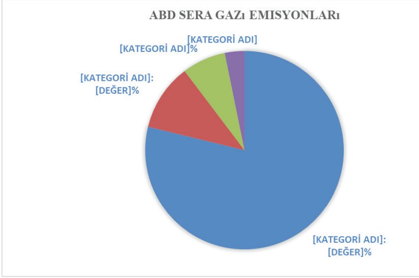
Şekil 2. ABD 2020 Yılı Sera Gazı Emisyonları (Kaynak: EPA, 2022b)
