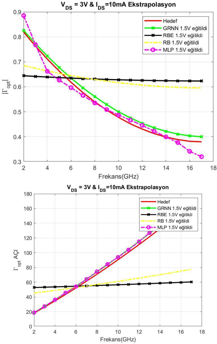
Şekil 2.4 Frekans ile |\Gamma_{opt}| ve \varphi_{opt} (açı) değişimi
