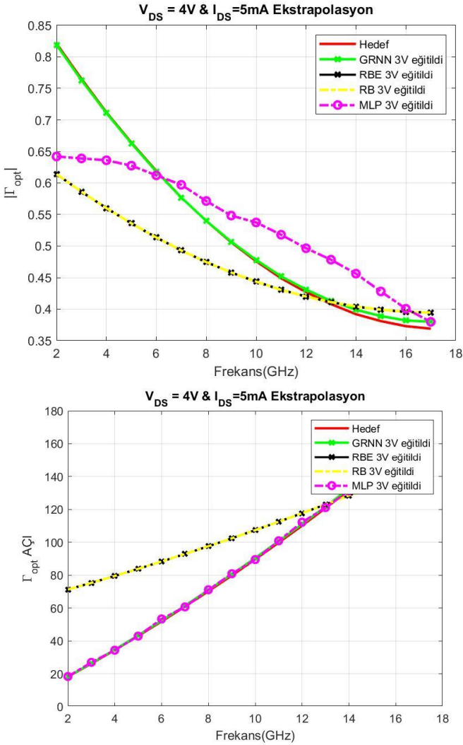
Şekil 2.18 Frekans ile |\Gamma_{opt}| ve \varphi_{opt} (açı) değişimi
