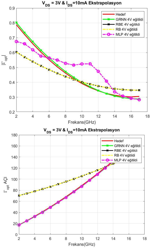
Şekil 2.24 Frekans ile |\Gamma_{opt}| ve \varphi_{opt} (açı) değişimi
