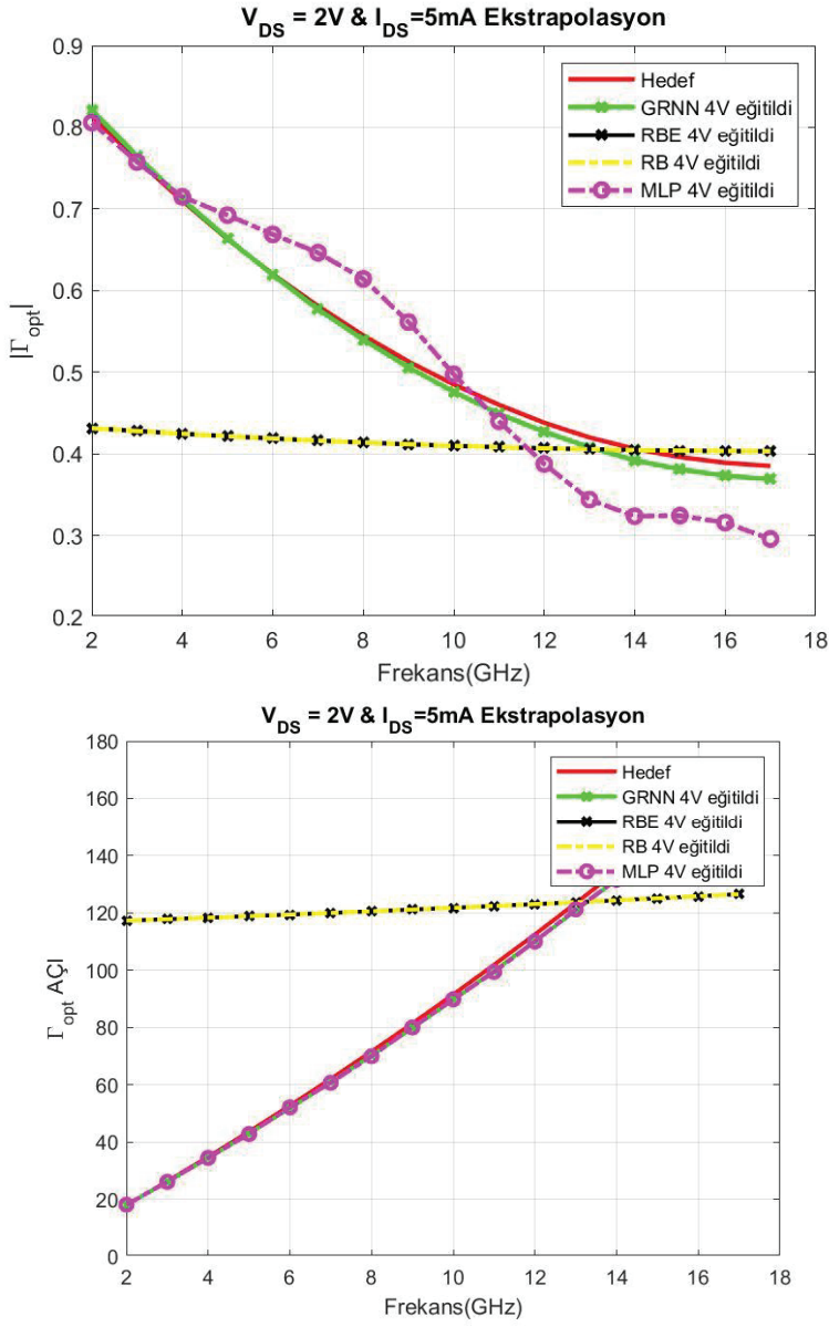
Şekil 2.22 Frekans ile |\Gamma_{opt}| ve \phi_{opt} (açı) değişimi
