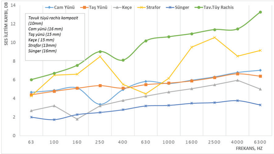
Şekil 5. Bazı geleneksel ses yalıtım malzemelerinin frekansa bağlı olarak ses iletim kaybı eğrileri
