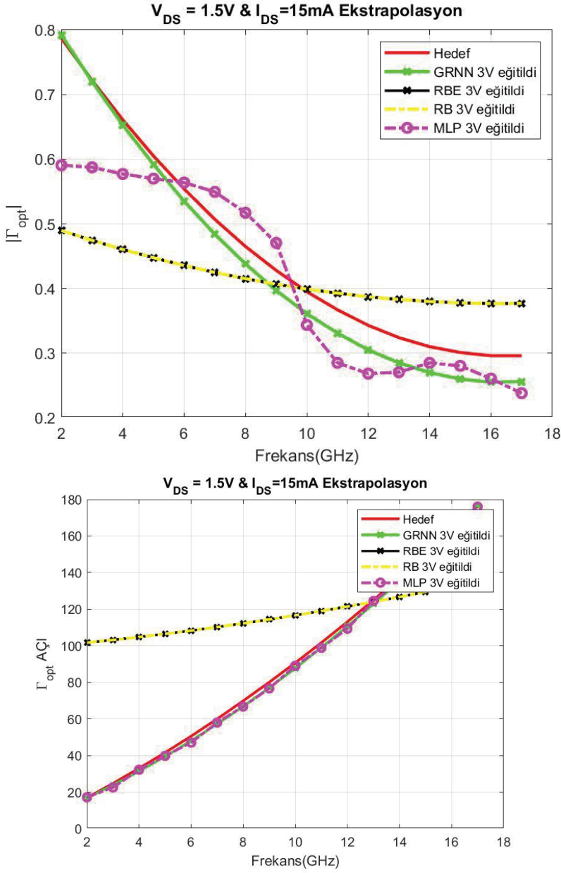
Şekil 2.14 Frekans ile |\Gamma_{opt}| ve \varphi_{opt} (açı) değişimi
