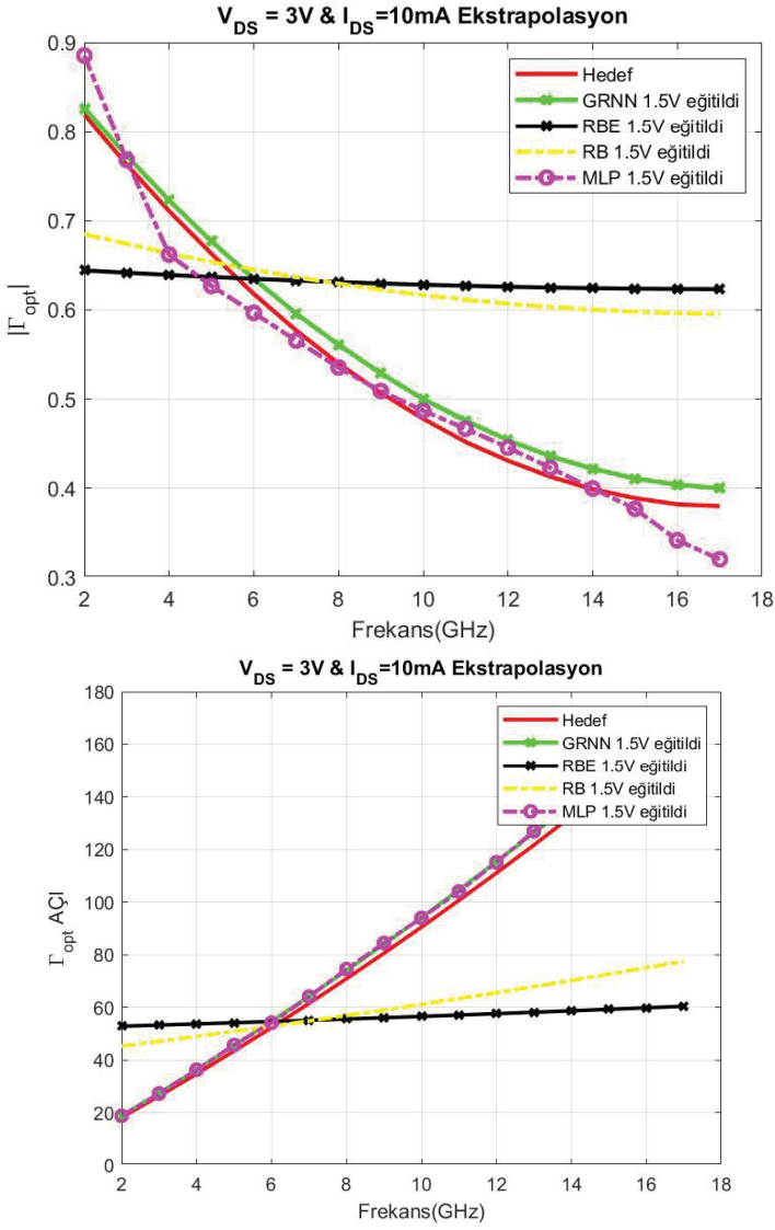
Şekil 2.4 Frekans ile |\Gamma_{opt}| ve \phi_{opt} (açı) değişimi
