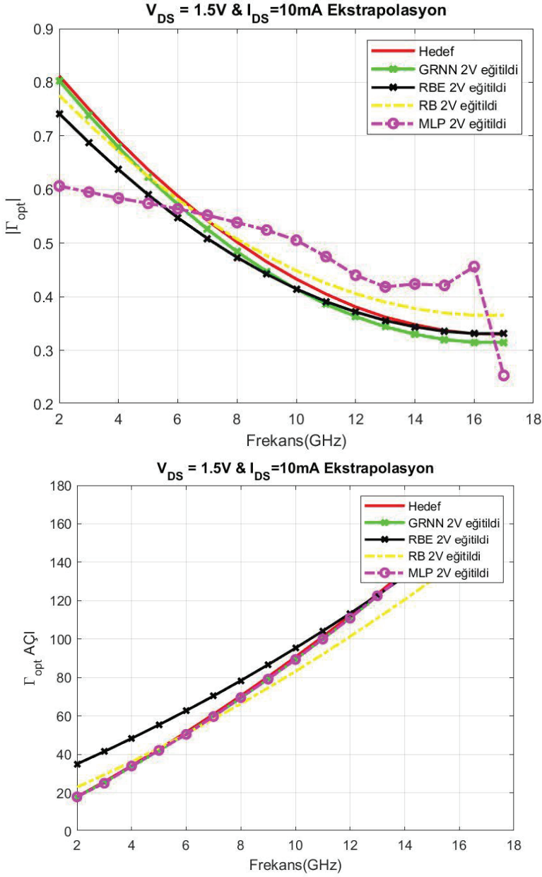
Şekil 2.8 Frekans ile |\Gamma_{opt}| ve \phi_{opt} (açı) değişimi
