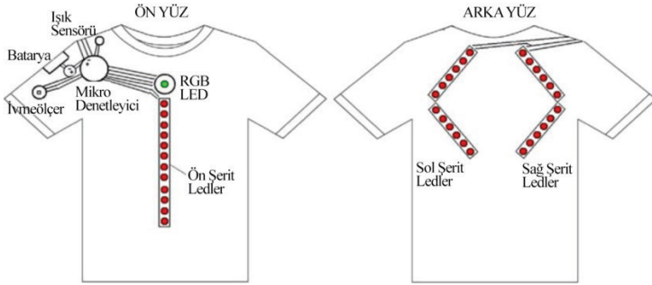
Şekil 4. Aktif tişört (Şenol, 2011)
