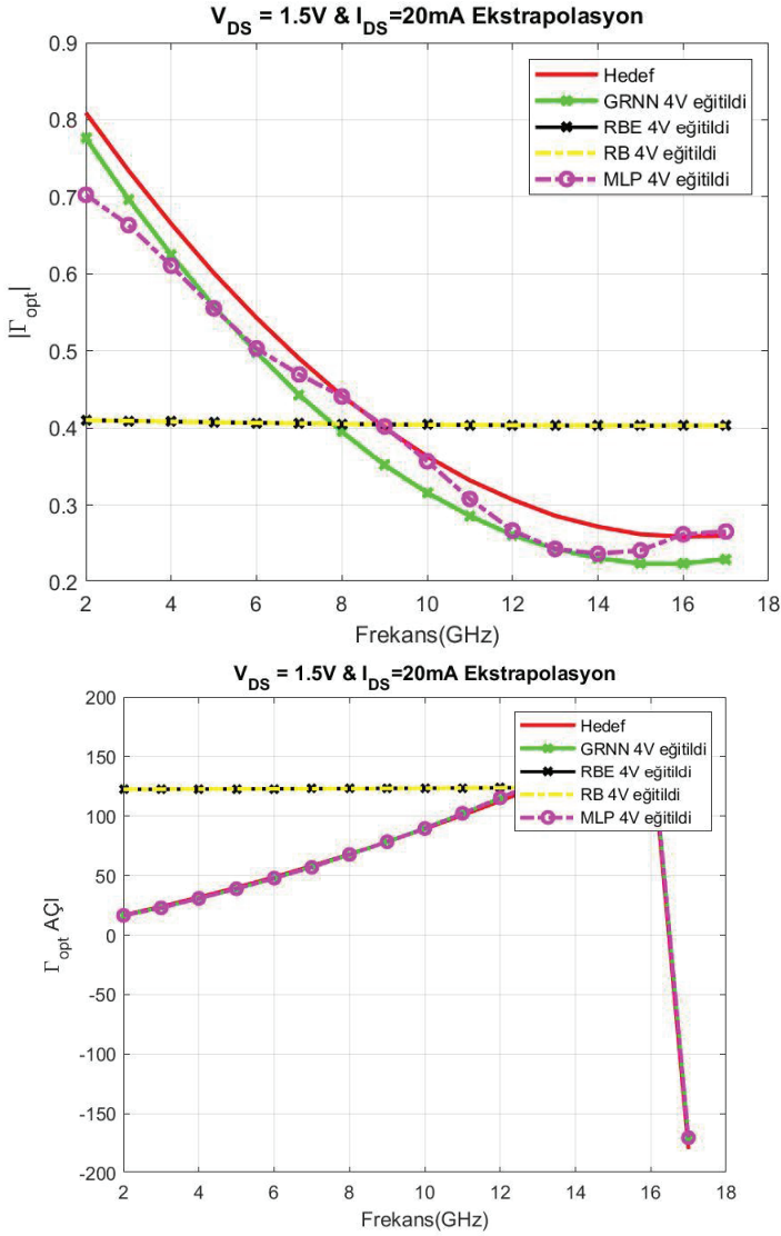
Şekil 2.20 Frekans ile |\Gamma_{opt}| ve \phi_{opt} (açı) değişimi
