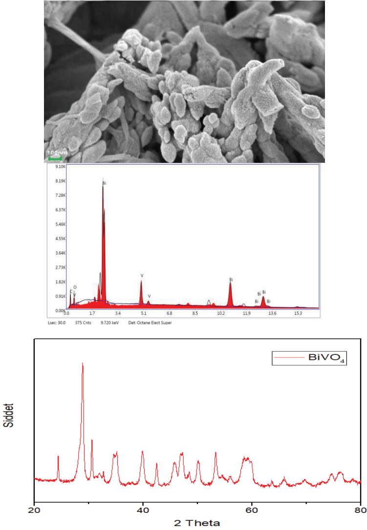
Şekil 7: Laboratuvarımızda üretilen \text{BiVO}_4 tozunun SEM, EDX ve XRD analiz sonuçları.
