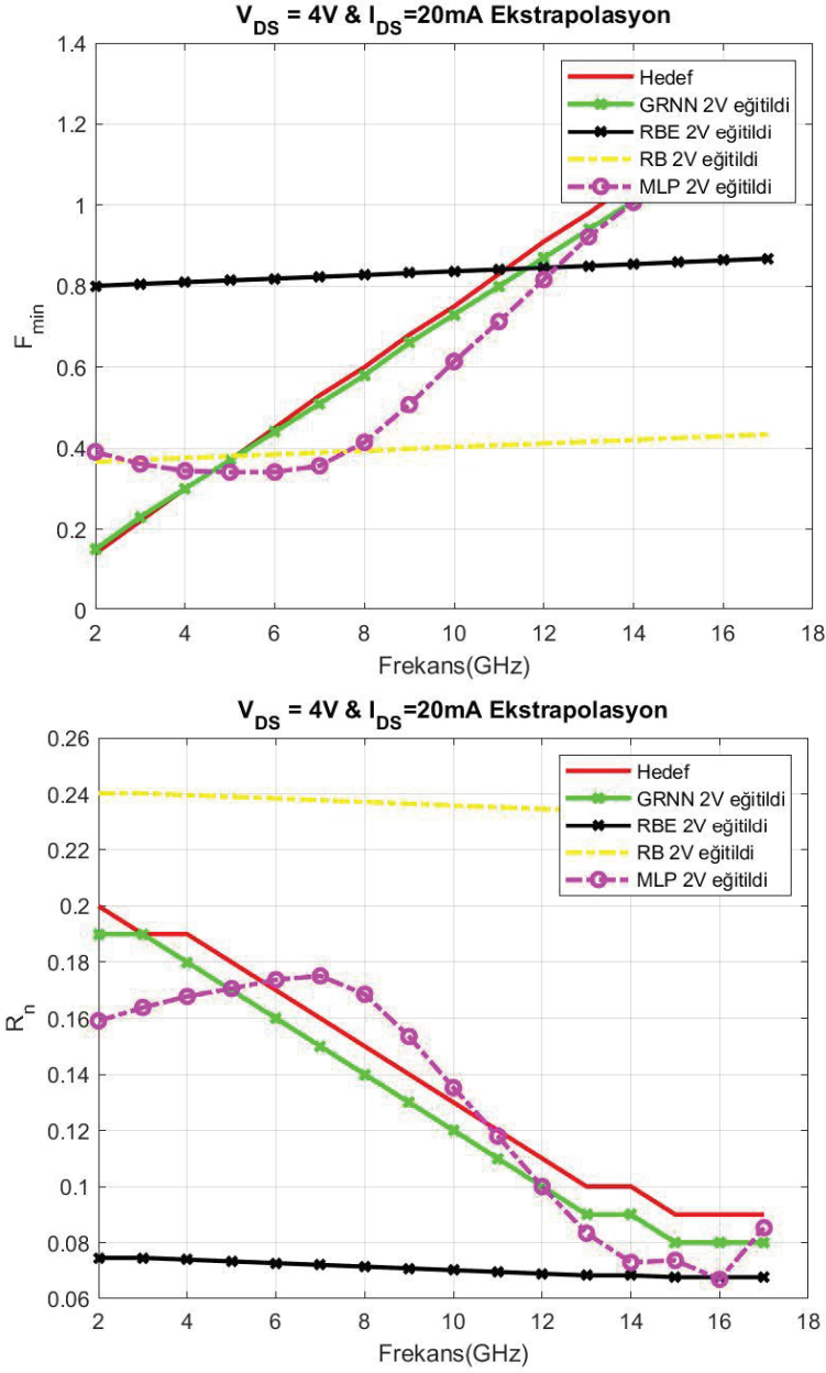
Şekil 2.11 Frekans ile F_{min} ve R_n / 50 değişimi
