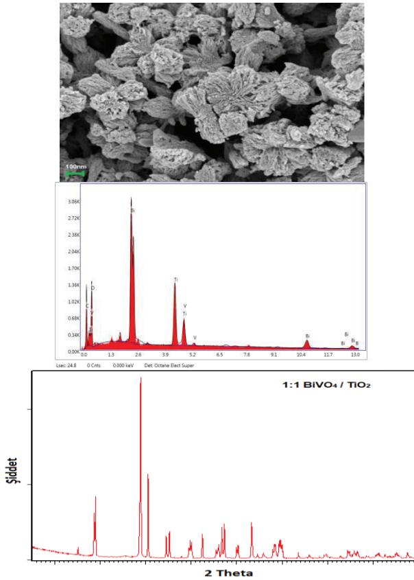
Şekil 8: Sentezlenen ve kalsine edilmiş 1:1 \text{BiVO}_4/\text{TiO}_2 nanofiber SEM, EDX ve XRD analizi.
