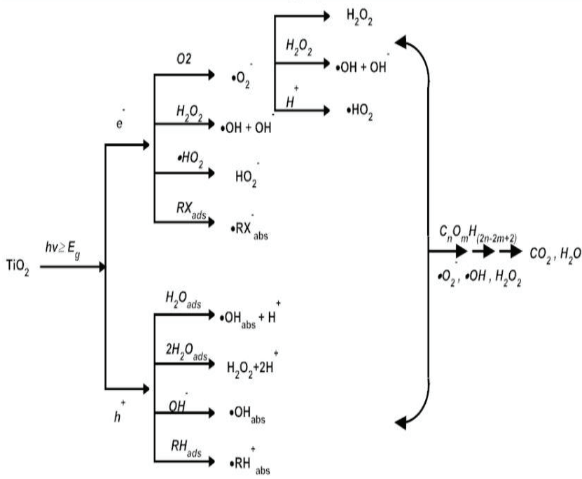
Şekil 4:Fotoelektrokimyasal mekanizmada üretim aktif oksijen türlerinde yer alan reaksiyon zinciri. Langenhove ve arkadaşlarından uyarlanmış, 2007 [44].
