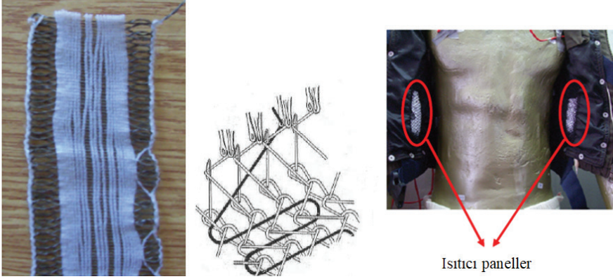
Şekil 6. Tekstil temelli ısıtıcı panel, örgülü örme yapısı, ısıtıcı giysi (soldan sağa) (Kayacan, 2008)
