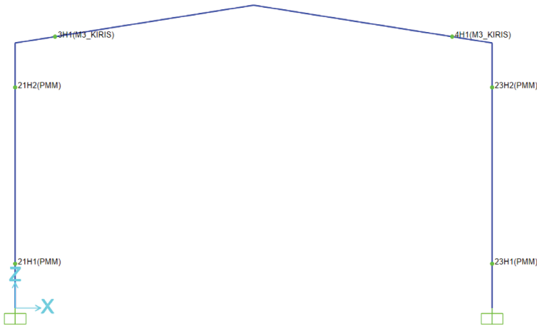
Şekil 4. SAP2000 Yazılımında Kolon Ve Kirişlere Atanan Mafsallar.
