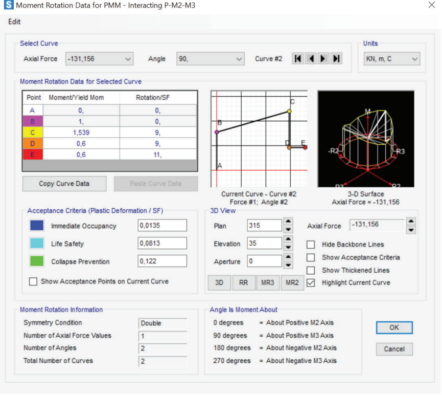
Şekil 7. SAP2000'de Kolon M2 Yönü Mafsal Özellikleri.
