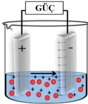
Şekil 1. EPD sistemi gösterimi (Batool et al., 2021)
