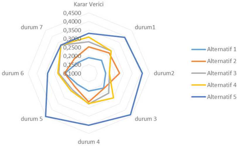
Şekil 7.1 VIKOR Yöntemi Q Değeri Duyarlılık Radar Grafiği
