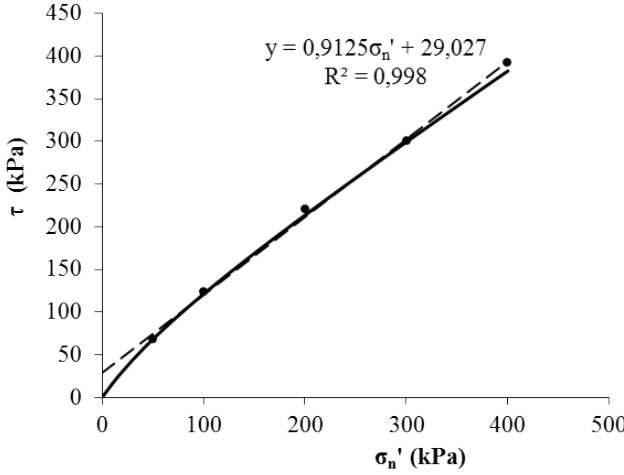
Şekil 12. Efektif normal gerilme ve kayma gerilmesi ilişkisi
