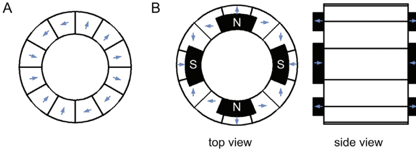
Şekil 3. Manyetik ilaç hedeflemede kullanılan dairesel Halbach dizisi örnekleri (Munoz et al., 2016; Riegler et al., 2011).
