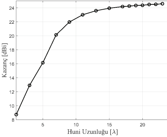
Şekil 9. Huni uzunluğunun ( R ) kazanca olan etkisi
