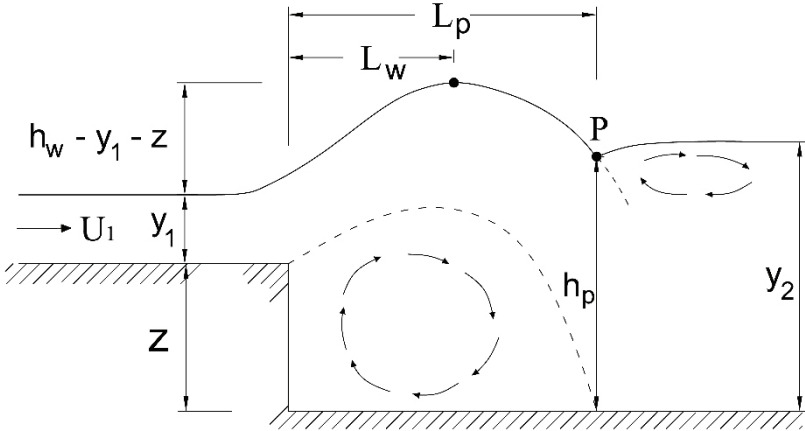
Şekil 3. Ani Taban Düşülerinde Oluşan Dalga Tipi Akımların Şematik Gösterimi Gözlemler
