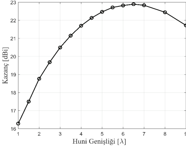
Şekil 7. Huni genişliğinin (A) kazanca olan etkisi
