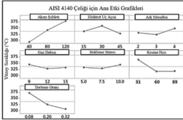
Şekil 9. İşlem parametrelerinin yüzey sıcaklığı üzerine etkileri
