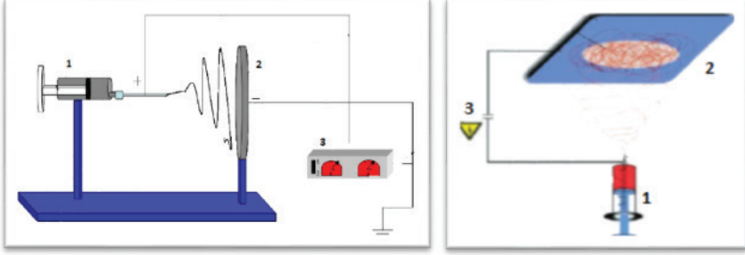
Şekil 3. Yatay (solda) ve Dikey (sağda) Elektroegirme düzeneği basit gösterimi (1: Besleme çözeltisi; 2: Toplayıcı plaka; 3: Yüksek voltaj; Kaynak: Kozanoğlu, 2006)
