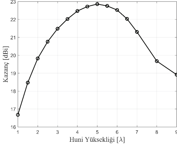
Şekil 8. Huni uzunluğunun (B) kazanç olan etkisi
