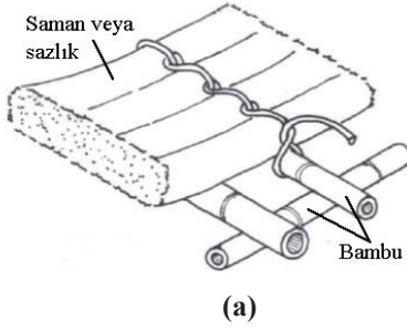
Şekil 12: Saman veya sazlık ile oluşturulan bambu çatı kaplaması a: (López, 2003), b: (URL-7).
