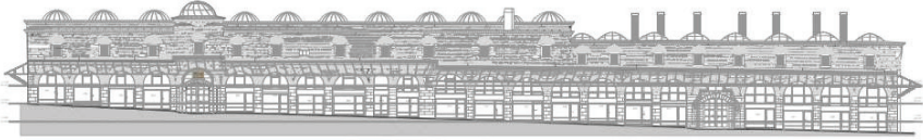
Şekil 20: Rüstempaşa Kervansarayı III. Dönem Cephe Restitüsyonu (Zağra, 2022)
