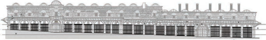
Şekil 16: Rüstempaşa Kervansarayı I.Dönem Cephe Restitüsyonu ( Zağra, 2022)
