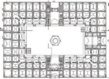
Şekil 8. Diyarbakır Hasan Paşa Han Planı (Özkarıcı, 1995)
