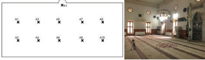
Şekil 5. Attar Ece Hoca Cami için kaynak (K1) ve alıcı noktalarının (A1, A2,..., A10) konumları
