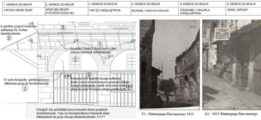
Şekil 10. Güvenilirlik Analizleri ve Detay Cephe Restitüsyonu (Zağra, 2022)
