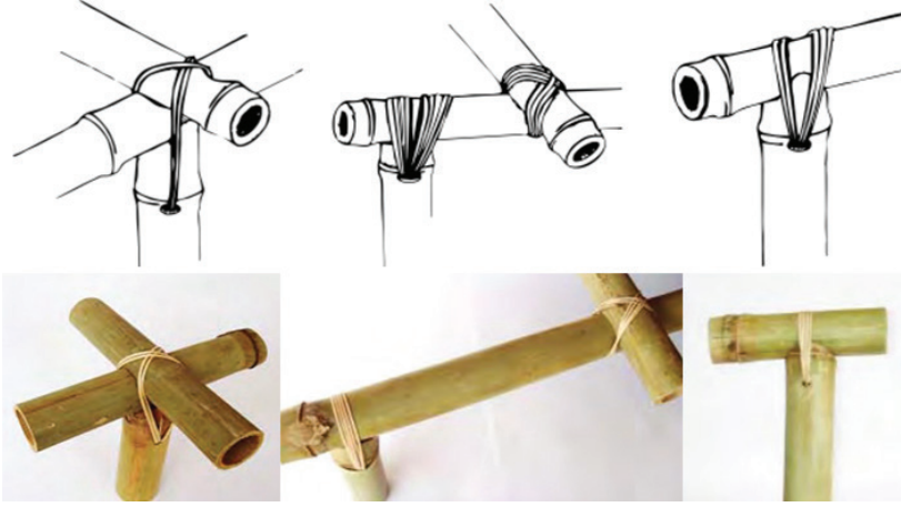
Şekil 20: Bambulara açılan deliklerden halat geçirilerek bağlama yöntemi (Reubens, 2010, s.130-131).
