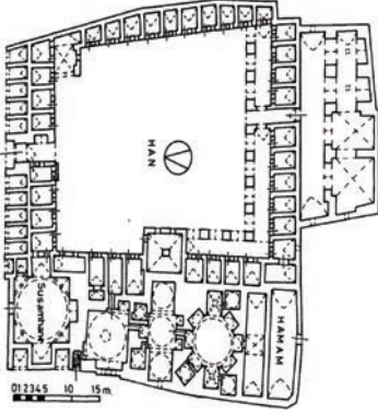
Şekil 6. Lala Mustafa Paşa Han Planı (Özkarıcı, 1998)
