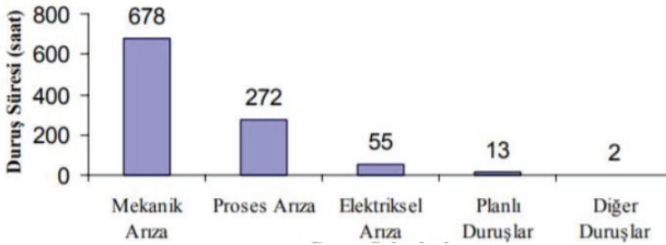
Şekil 8. Sivas Çimento Fabrikasındaki Makine Duruşlarının Pareto Grafiği
