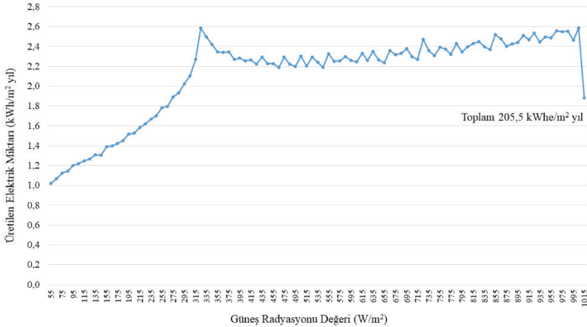
Şekil 9. Birim m²'ye elektrik üretiminin güneş radyasyonu ile değişimi
