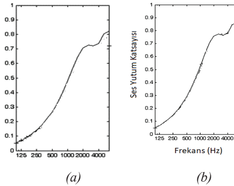
Şekil 13: (a) Jüt (b) yün liflerinin ses yutum performansları [44].
