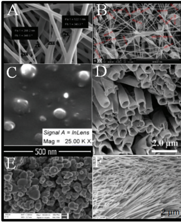
Şekil 7. SEM görüntüleri kaydedilen; A) sodyum aljinat içeren nanolifler (Ceylan ve ark., 2018c), B) nanoenkapsüle L. reuteri bakterileri (Ceylan ve ark., 2019b); C) buğday tohumu yağı içeren nanoemülsiyonlar (Ceylan ve ark., 2019a); D) bovin serum albümin+ \kappa -karragenan nanotüpleri (Maldonado ve ark., 2019); E) \text{TiO}_2 tozlarının nanoyapısı (Dazon ve ark., 2019); F) ZNO nanotelleri (Zhou ve ark., 2006)
