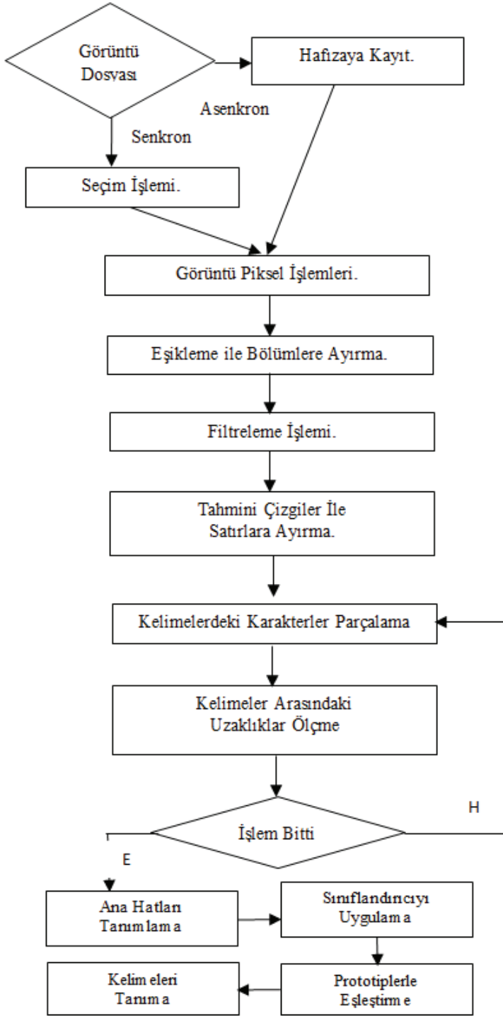
Şekil 1. Tesseract Çalışma Yapısı (Mithe ve ark.,2013)
