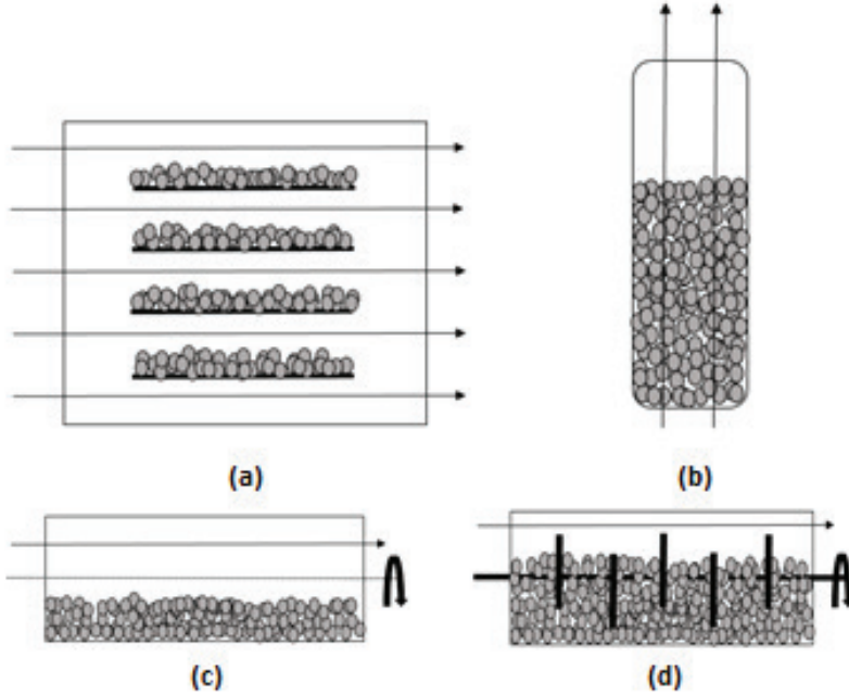
Şekil 1. Katı Kültür biyoreaktör tipleri: a) Tepsili b) Dolgulu kolon c) Döner tambur d) Karıştırılmalı tambur (oklar hava akış yönünü göstermektedir).
