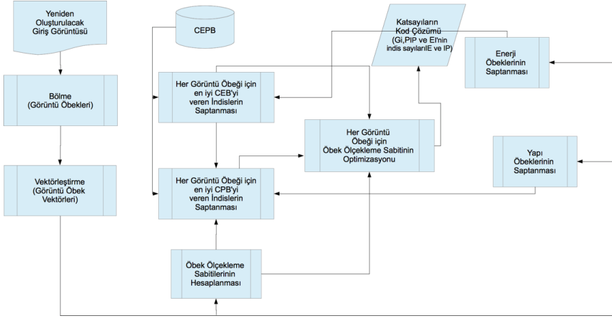
Şekil 4. Kodlama Süreci Akış Şeması (Verici Kısım Kodlama Süreci)
