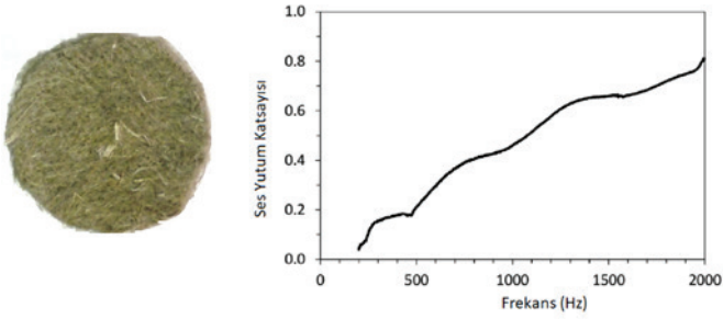
Şekil 9: Kenevir lifi ses yutum performansı (3 cm) [52].
