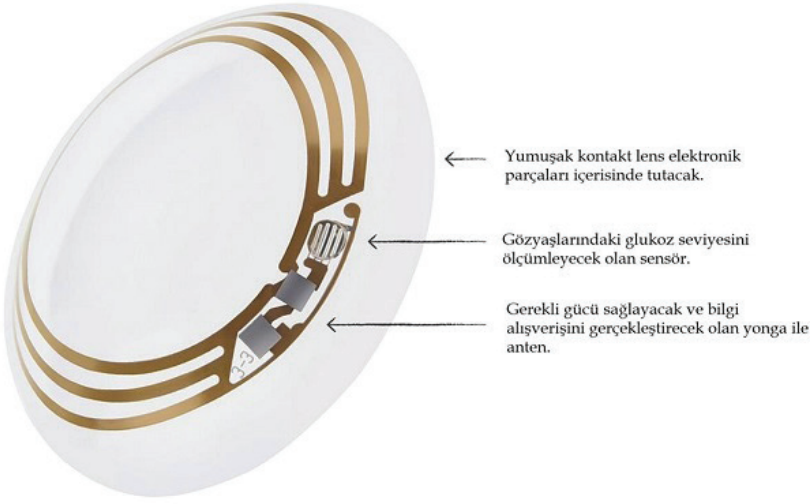
Şekil 3: Google Akıllı kontak Lens (Google'dan Akıllı Lens, 2017)
