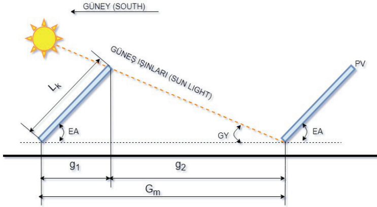
Şekil 7. Dizi halinde yerleştirilmiş kolektör arası mesafe hesabı
