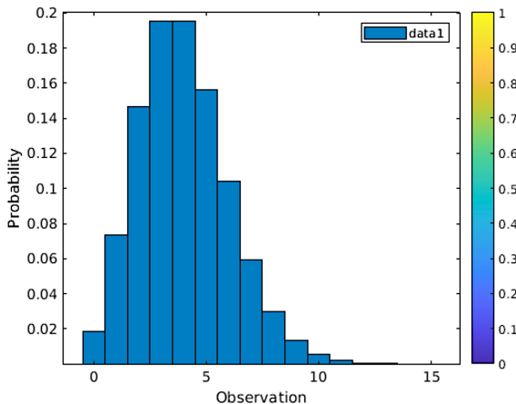
Şekil 1: Poisson Dağılımı
