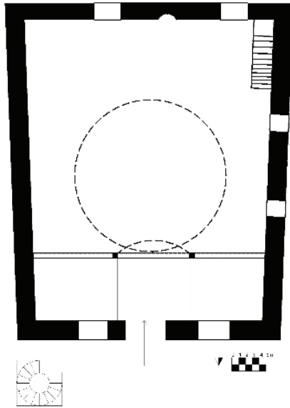
Çizim 1. Ahat Köyü Yukarı Cami (S.Erçin Koçer) 1
