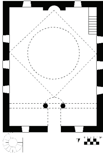
Çizim 2. Susuz Köyü Cami (S.Erçin KOÇER)
