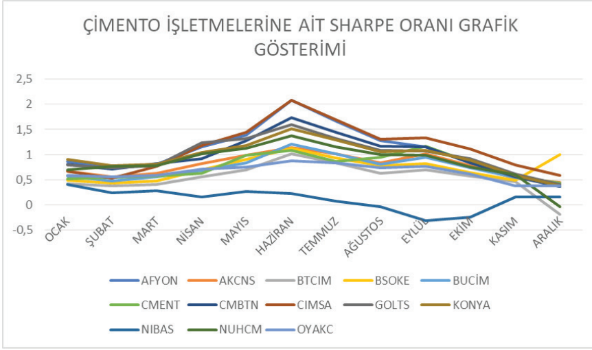
Şekil 1. Sharpe Oranı Uygulamasının Grafik Gösterimi
