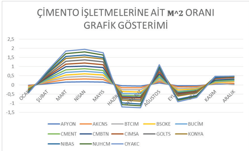
Şekil 2 . M^2 Oranı Uygulaması Grafik Gösterimi
