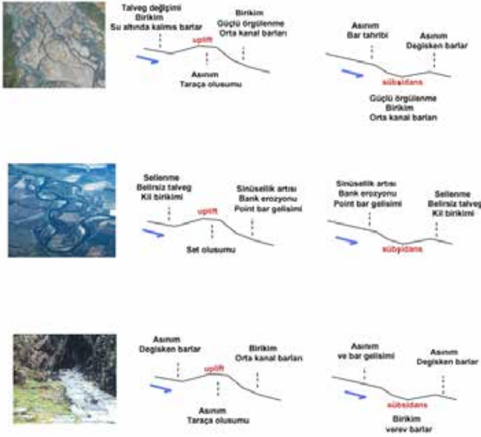
Şekil 11: Menderesli akarsu yataklarında uplift ve sübsidansa nehir tepkisi (Schumm vd., 2000'den değiştirilerek).
