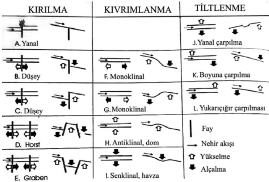
Şekil 1: Yeryüzünün deformasyon türleri (Schumm vd., 2000'den düzenlenerek).
