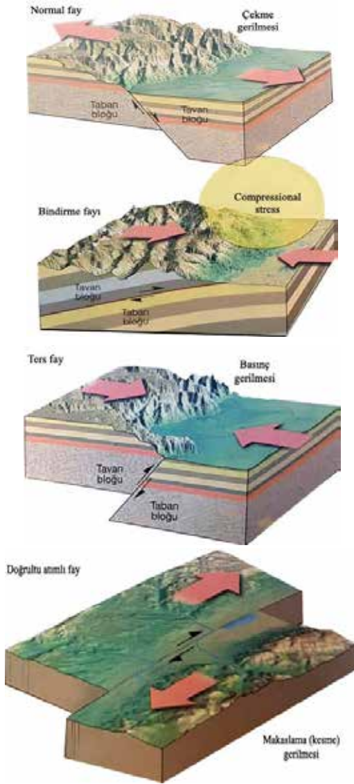
Şekil 3: (A) Fay türleri (Erinç, 2005). (B) Normal fay ve Bindirme fayının gelişimi. (C) Ters fay gelişimi. (D) Doğrultu atımlı fayın gelişimi (Helvacı, 2013).
