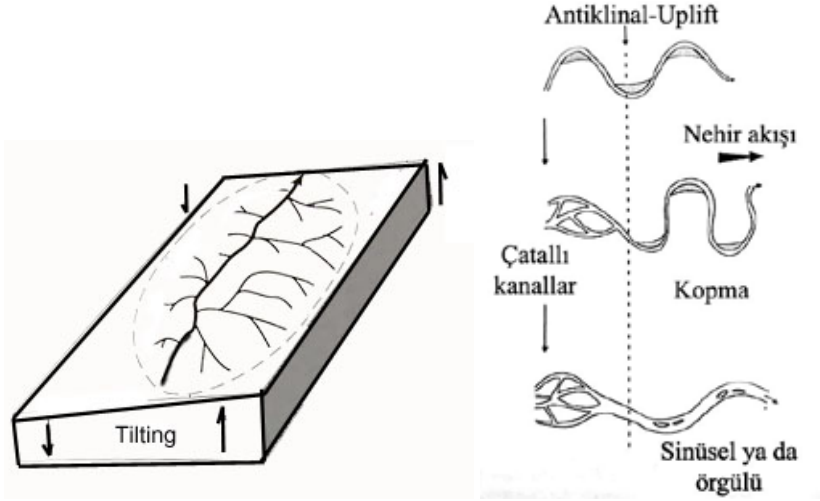
Şekil 2: (A) Tektonik çarpılmanın sebep olduğu asimetrik drenaj gelişimi ( Killer ve Pinter, 2002 ). (B) Ani kanal paterni değişimi ( Schumm, 1977 ).
