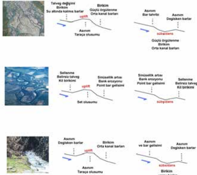
Şekil 10: Örgülü akarsu yataklarında uplift ve sübsidansa nehir tepkisi (Schumm vd., 2000'den değiştirilerek).
