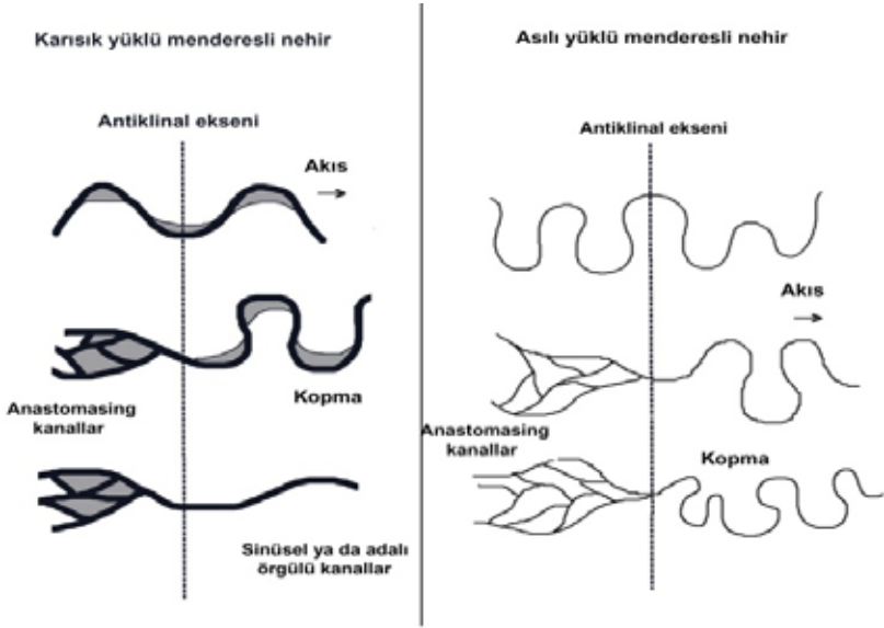
Şekil 12: Menderesli bir nehrin sediment boyutuna göre upliftte tepkisi (Schum, 1977).
