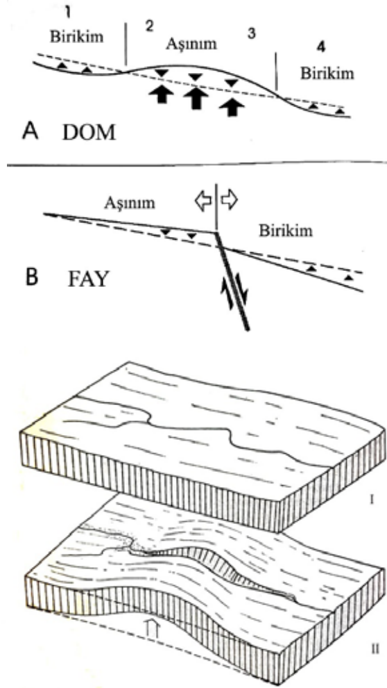
Şekil 7: (A, B) Uplift ve lokal faylanma ile gelişen aşınım ve birikim lokasyonları (Schumm vd., 2000'den düzenlenerek). C. Antesedant vadi gelişimi (Erinç, 2005).
