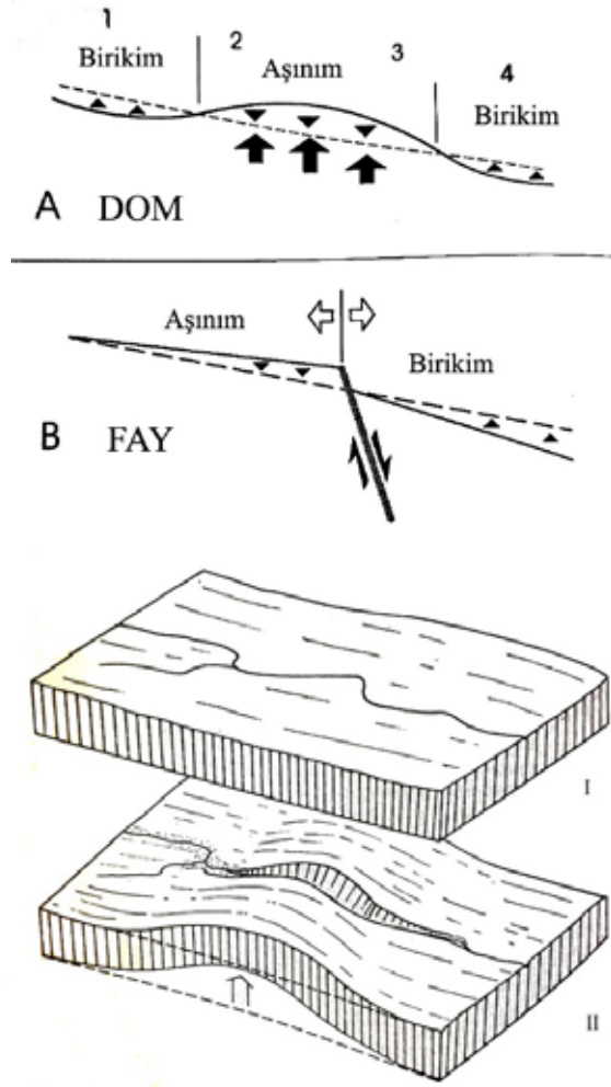
Şekil 7: (A, B) Uplift ve lokal faylanma ile gelişen aşınım ve birikim lokasyonları (Schumm vd., 2000'den düzenlenerek). C. Antesedant vadi gelişimi (Erinç, 2005).
