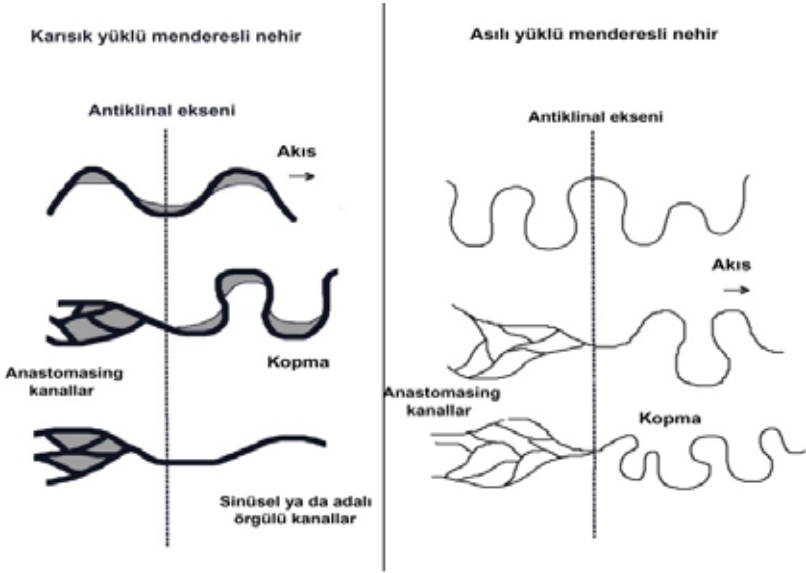
řekil 12: Menderesli bir nehrin sediment boyutuna gȳre upliftte tepkisi (Schum, 1977).
