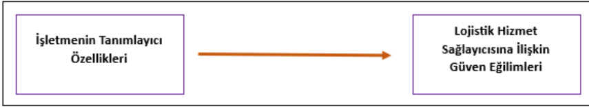
Şekil 1. Araştırmanın Modeli
