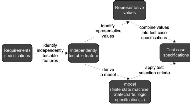
Şekil 6. Sistematik Stres Testi Akış Şeması (Kaynak: Baresi, 2016)
