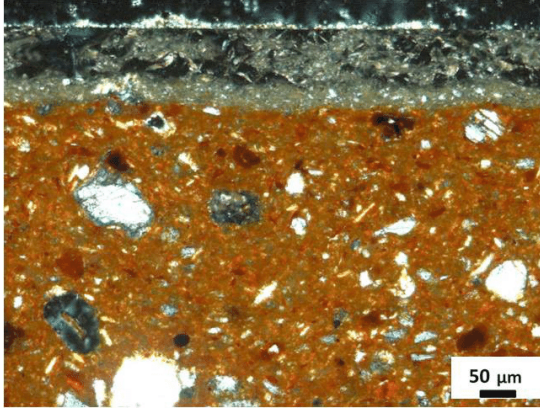
Resim 4: Tipik bir seramik örneğine ait ince kesit. Sır katmanı ve çeşitli minerallerden oluşan seramik hamuru görülmektedir (Rovella vd., 2019).
