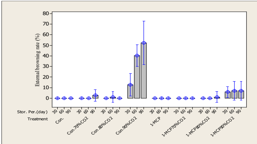
Şekil 3. “Hachiya” Trabzon hurması çeşidinde 1-MCP ve CO 2 uygulamalarının 90 gün depolanan meyvelerde yüksek karbondioksit zararı oranına etkisi (%)
