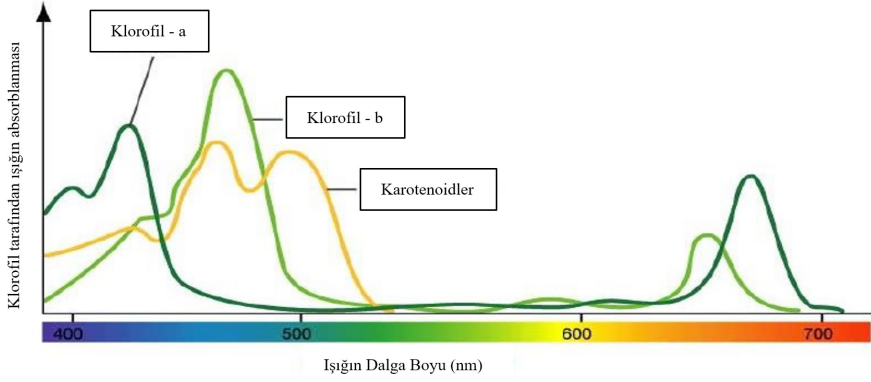
Şekil 2. Farklı dalga boylarının, farklı klorofil pigmentleri tarafından absorbe edilmesi (Khanacademy, 2020)
