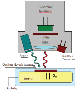
Şekil 7. Floresan bazlı gaz sensörü (Gök, 2007)
