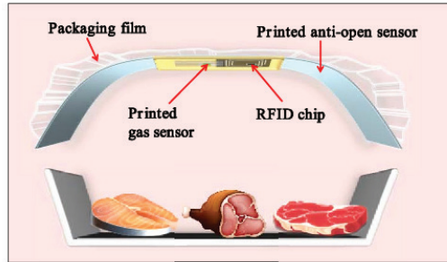
Şekil 10. RFID etiket ve gaz sensör entegrasyonu
